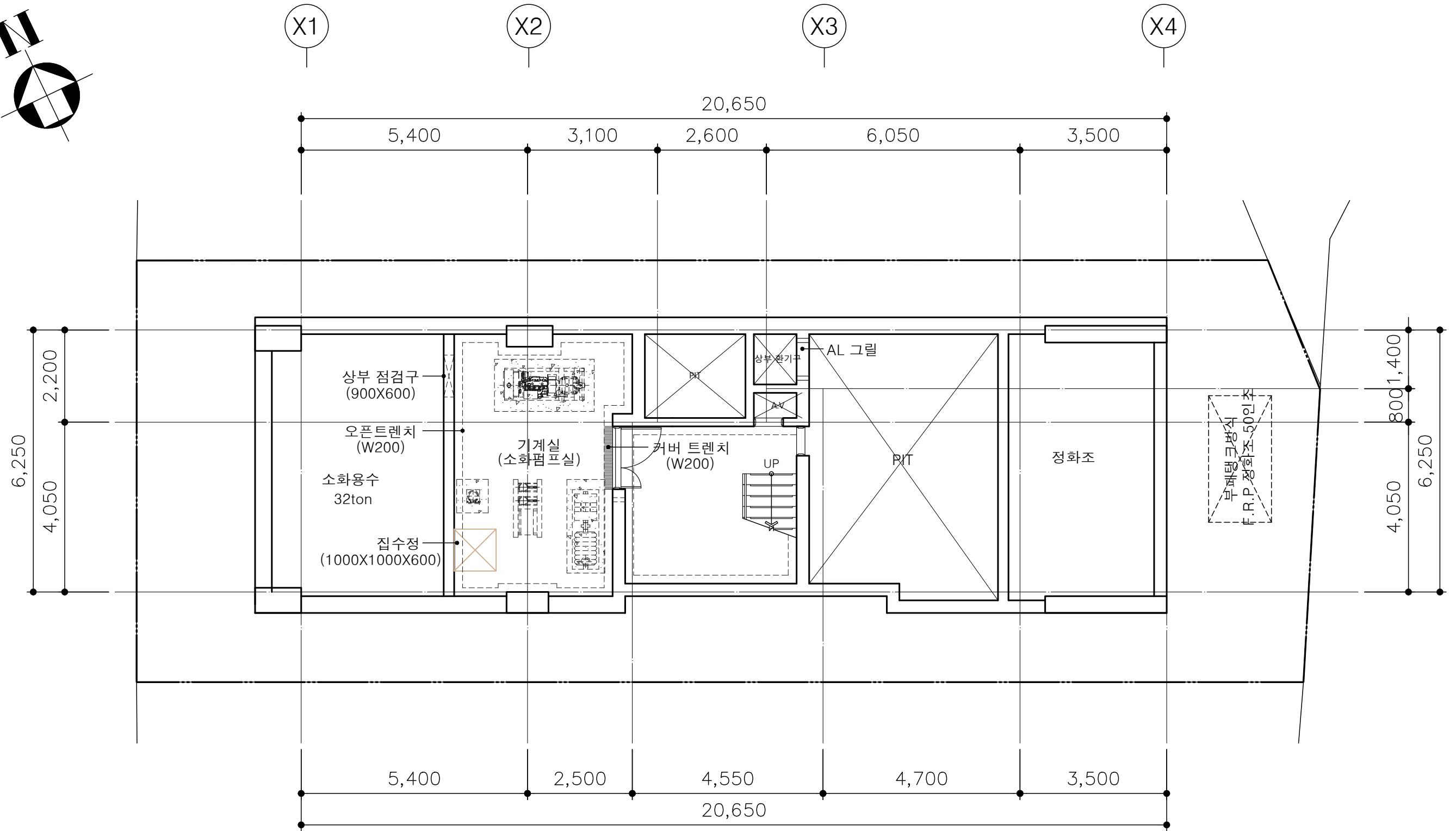
지하1층 평면도 축척:1/100
